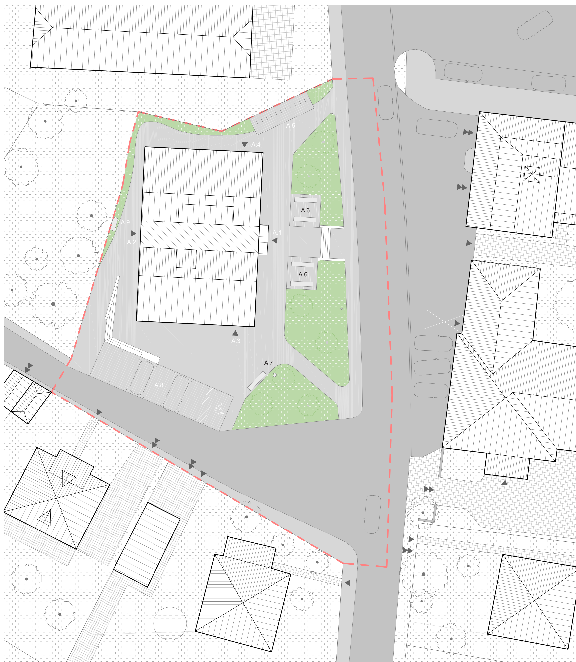
Situace | 1:250
